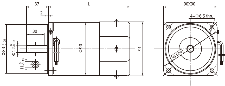
图11 90YS60 ( 60W ) 交流三相电机, 长度L=123mm ) ; 90YS60 ( 60W ) Three-Phase AC Motor, Length=123mm ) 90YS90 ( 90W ) 交流三相电机, 长度L=138mm ) ; 90YS90 ( 90W ) Three-Phase AC Motor, Length=138mm )
